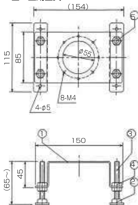
■ 2型用金具
