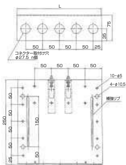
ヘッダパネル (シングル)
