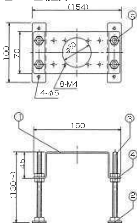
■ 1・3型用金具
