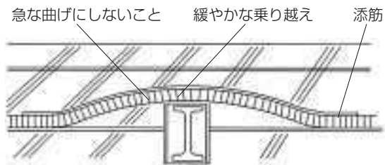
梁伏せ越し部
